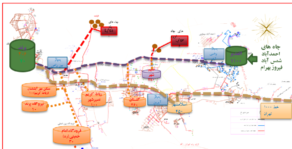
تصویر (۳-۱) سیمای تامین و انتقال آب به بهارستان
